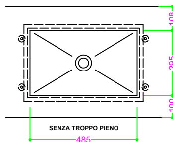
PROF. 503 senza foro rubinetto
