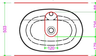
Foratura nel top PROF. 503
