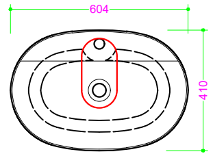
Vista Superiore
