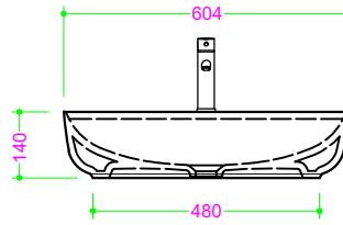
Vista Frontale
