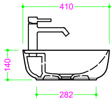
Sezione Longitudinale
