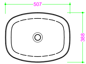
Vista Superiore
