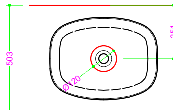
Foratura nel top PROF. 503 senza foro rubinetto
