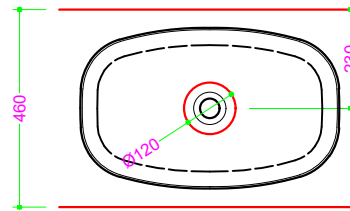
Foratura nel top PROF. 460 senza foro rubinetto
