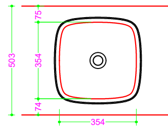
Foratura nel top PROF. 503 senza foro rubinetto
