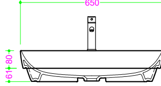
Vista Frontale
