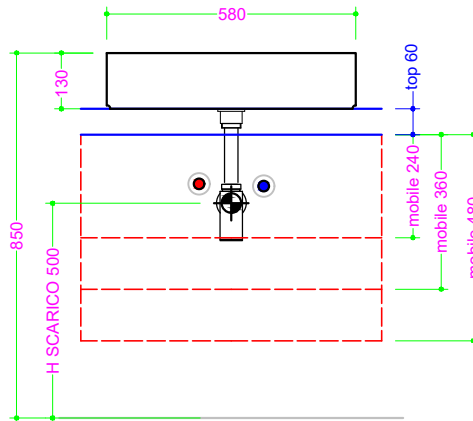
Foratura nel top PROF. 333 senza foro rubinetto
