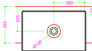
Foratura nel top PROF. 333 senza foro rubinetto
