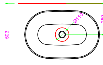
Foratura nel top PROF. 503 senza foro rubinetto
