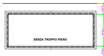
PROF. 503 senza foro rubinetto
