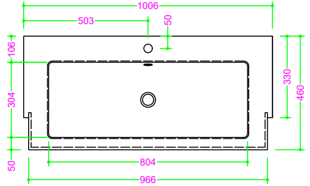
Vista Superiore
